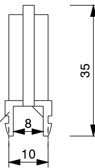
Halterung für in Rohr-C-Schiene (RC)
